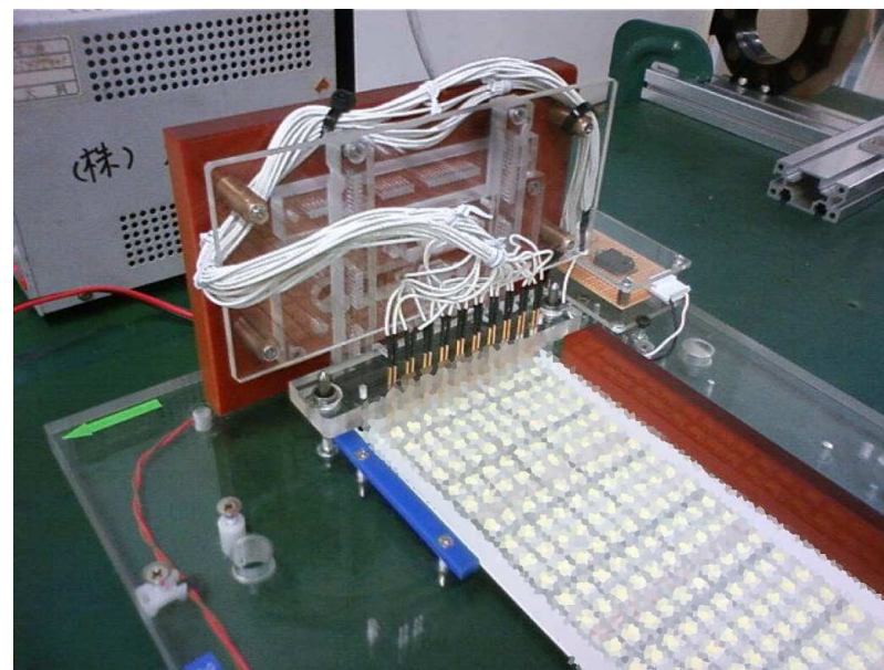
LED点灯検査冶具
